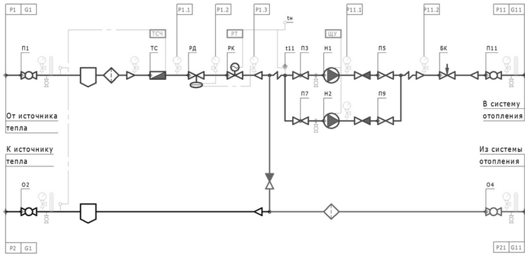
Зависимая схема с двухходовым клапаном и насосами в подающем трубопроводе
