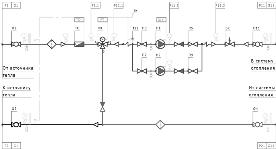
Зависимая схема с трехходовым клапаном и циркуляционными насосами
