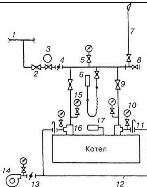
Схема обязательных газопроводов низкого давления котла, оборудованного горелками с принудительной подачей воздуха и отключающими устройствами — кранами
