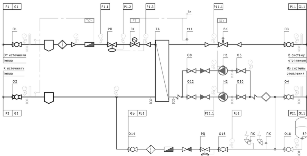
Зависимая схема с трехходовым клапаном и циркуляционными насосами
